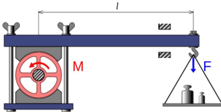
Slika 19. Pronijeva kočnica [18]
