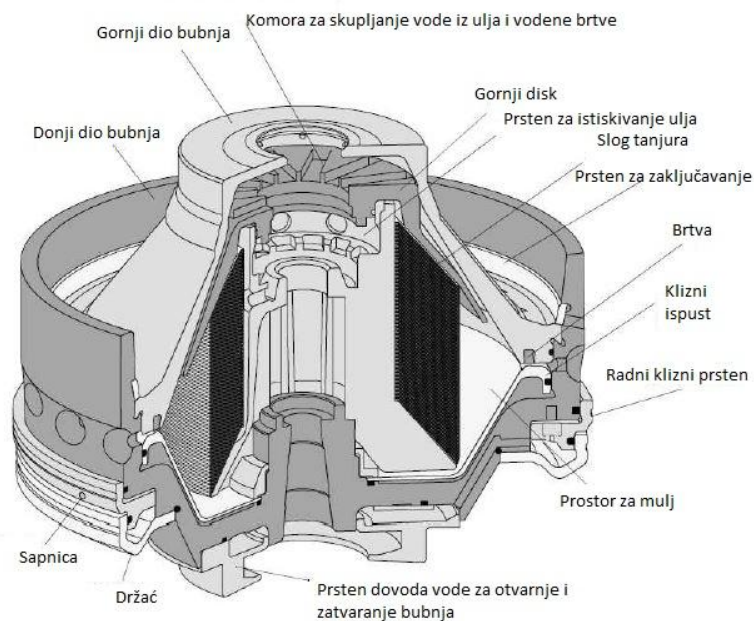
Slika 8. Bubanj centrifugalnog samočistioca sa sapnicom [8]
