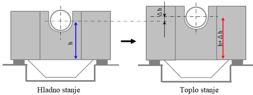
Slika 21. Vertikalni pomak središta ležaja uzrokovan temperaturnim širenjem temeljne ploče [2]
