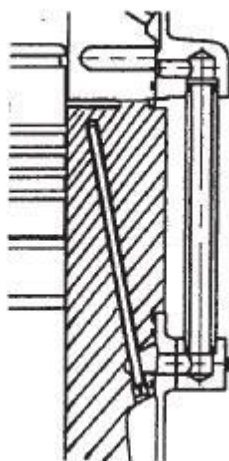
Slika 17. Novi dizajn provrtom hlađene košuljice [1]
