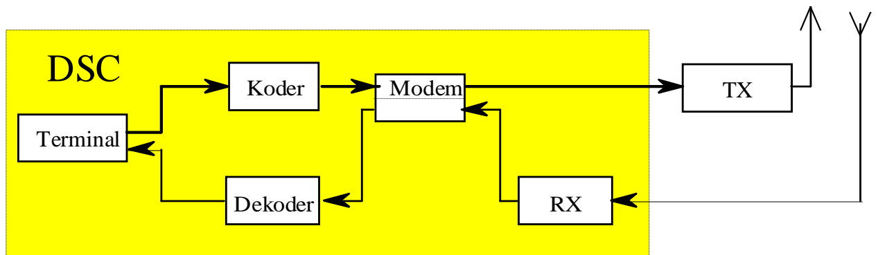
Slika 21. Blok shema DSC uređaja
