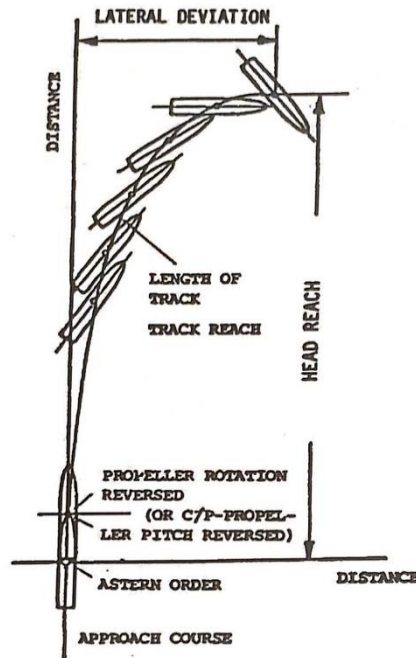
Slika 31. Pokus zaustavljanja
