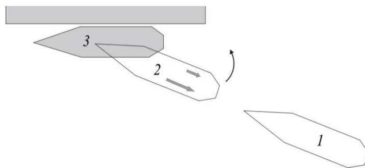
Slika 59. Uplovljenje brodom sa dva vijka
