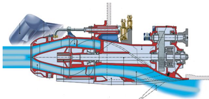
Slika 7. Vodomlazni propulzor
