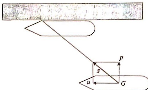
Slika 24. Djelovanje veznog konopa iz težišta broda
