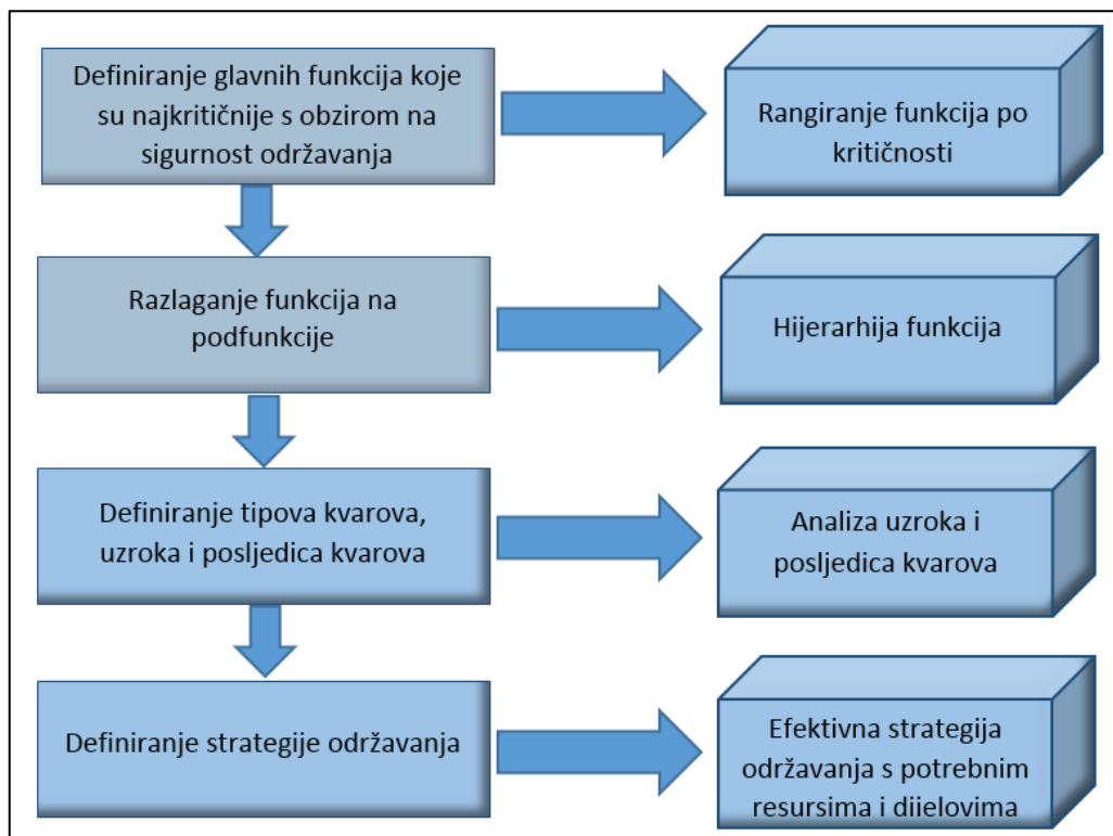
Slika 7. RCM metodologija
