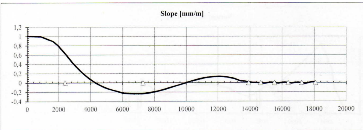
Slika 14. Graf nagiba uslijed nultih pomaka nosača [4]
