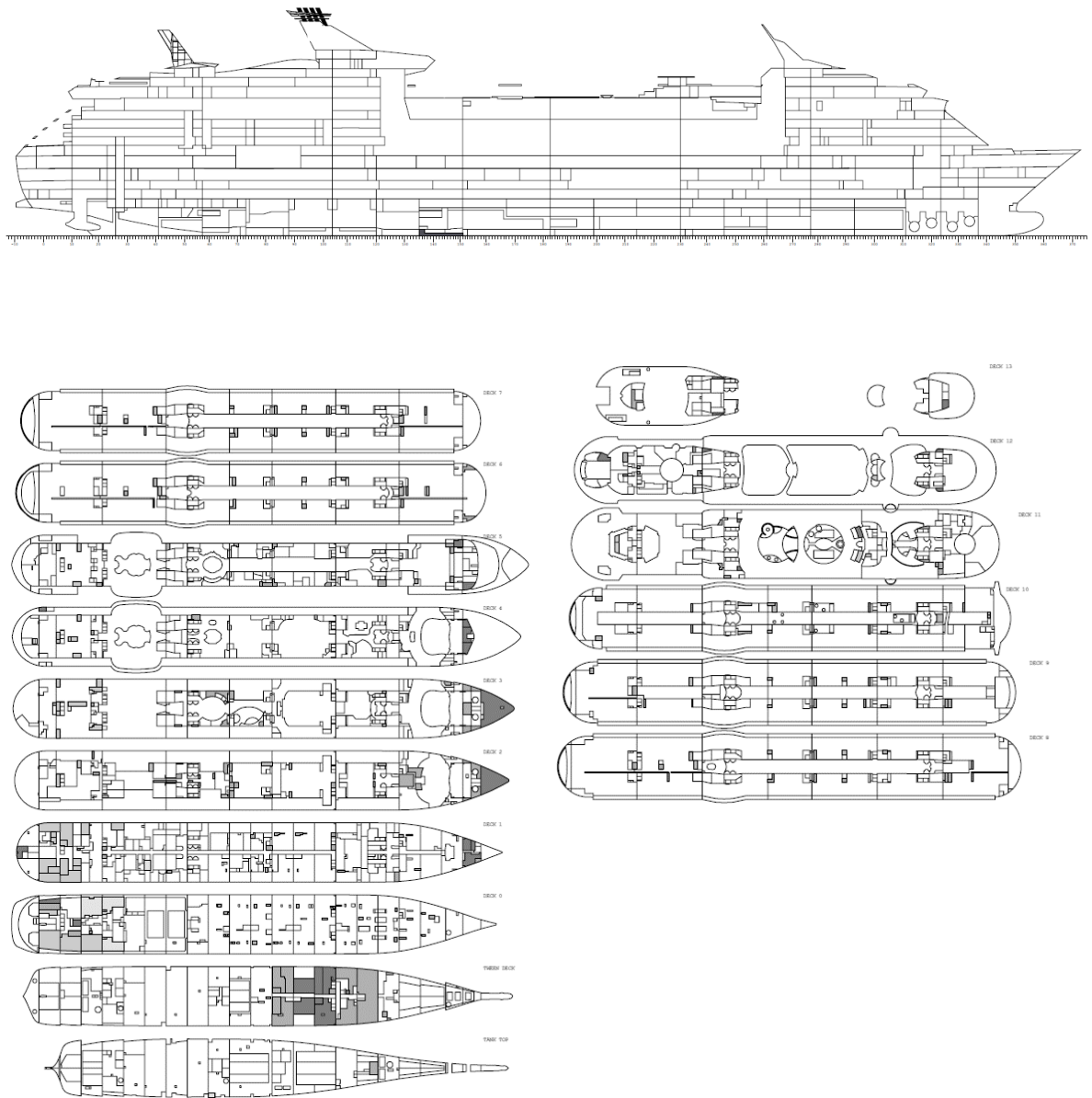
Slika 3: Isječak iz HT, generalni plan broda
