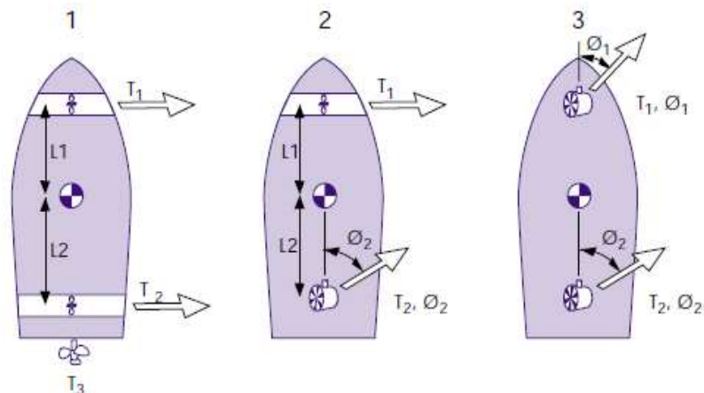
Slika 13. Minimalna propulzijska konfiguracija DP plovila [3]
