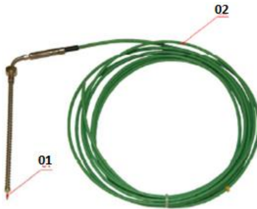
Slika 6. Termopar [11]
