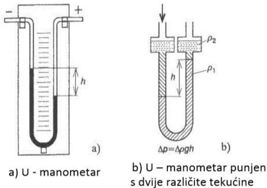
Slika 7. U-manometar [4]
