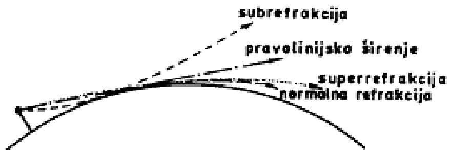
Slika 12. Utjecaj refrakcije na domet radara[6]
