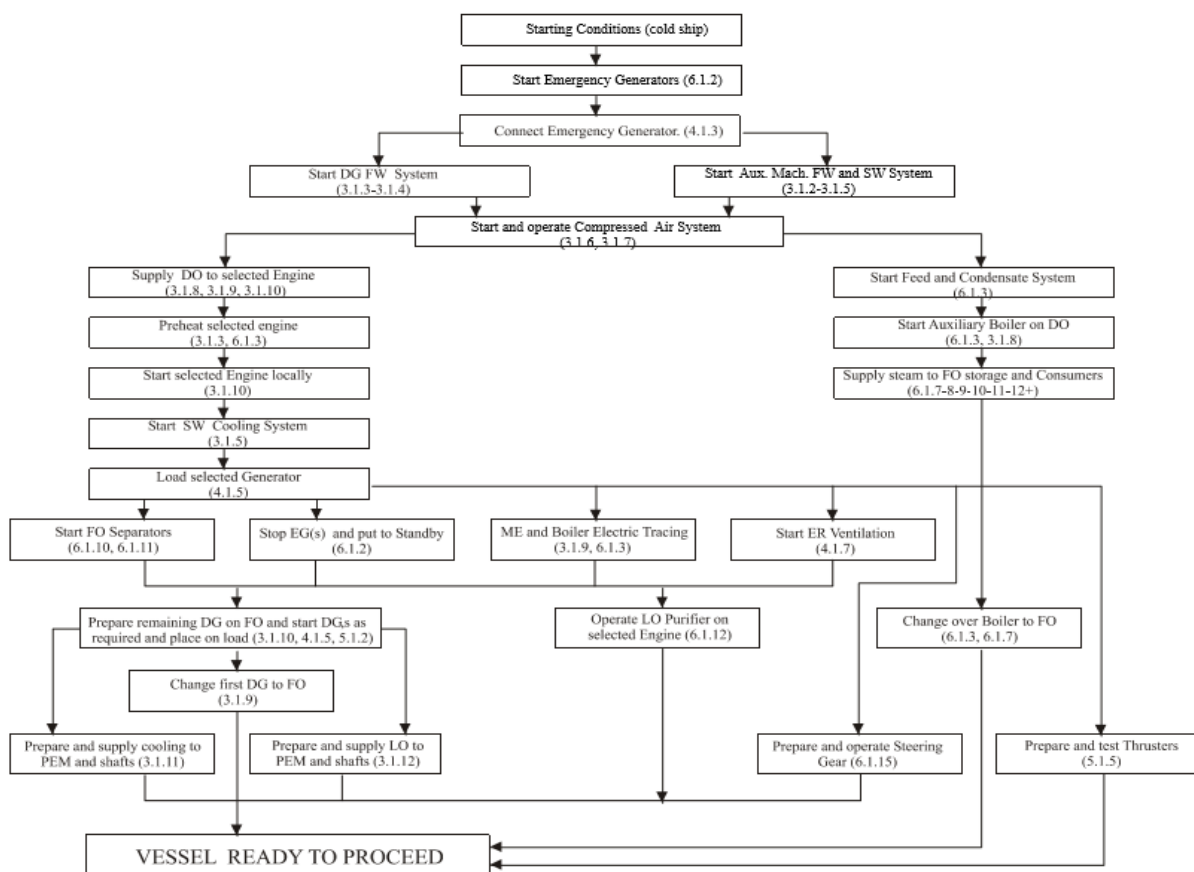
Slika 6. Slijedni dijagram toka [1]
