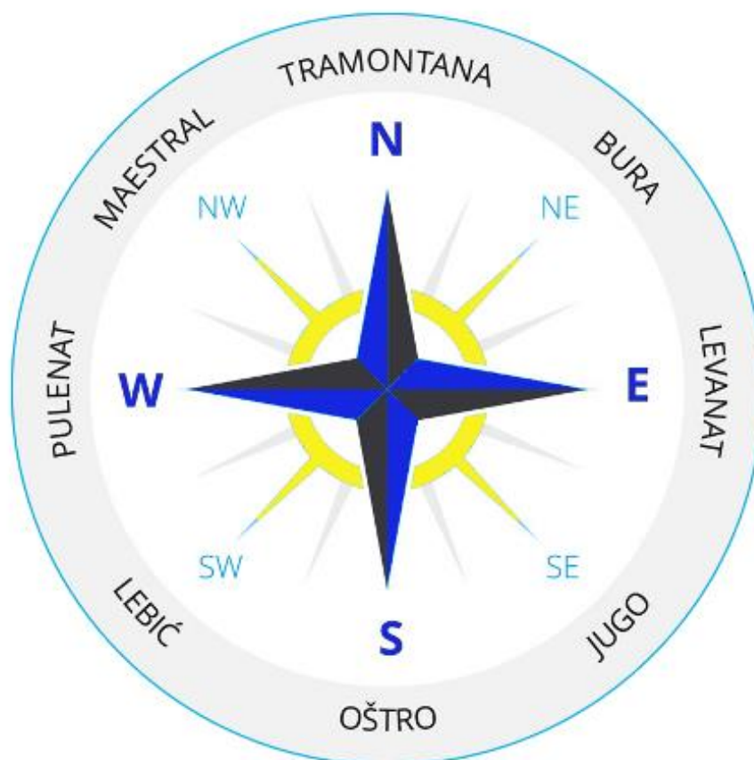
Slika 22- Ruža vjetrova [15]
