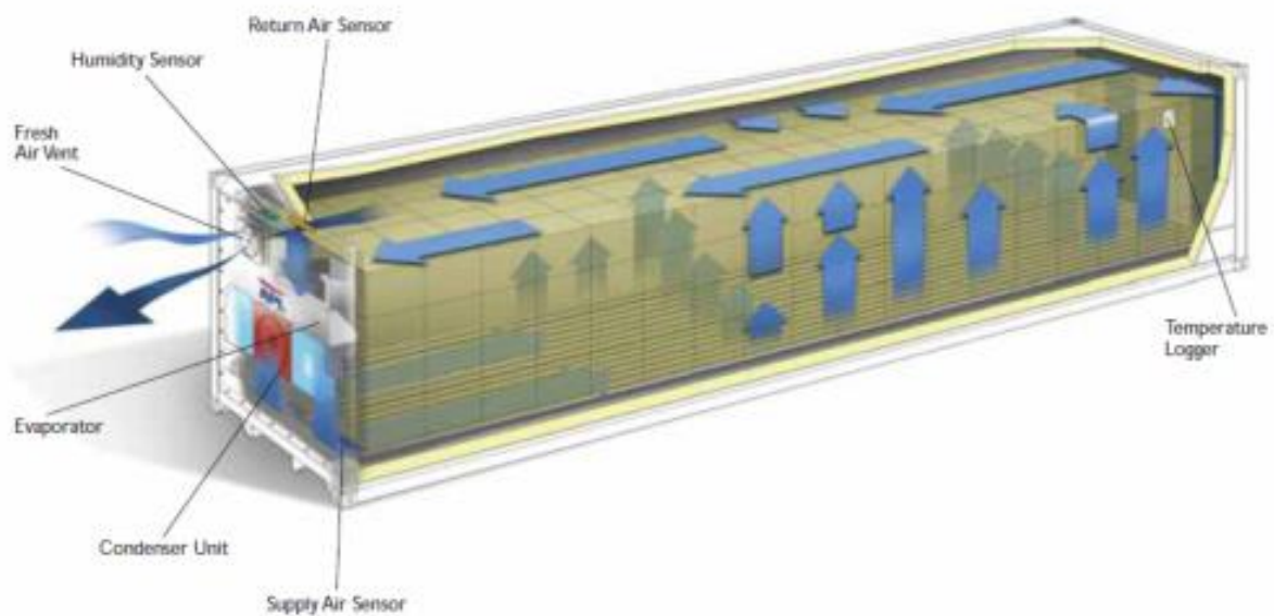
Slika 8. Rashladni kontejner
