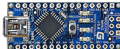
Slika 9. Arduino Nano
