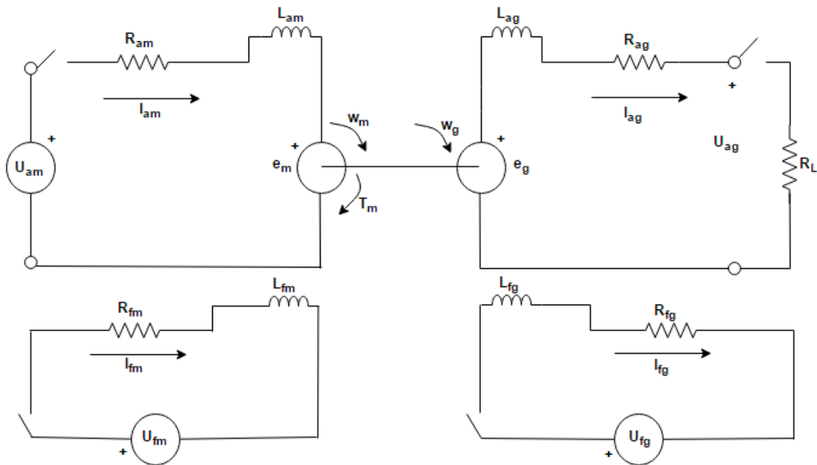
Slika 16. Načelna shema sprege istosmjernog električnog stroja motor-generator s nezavisnom uzбудom
