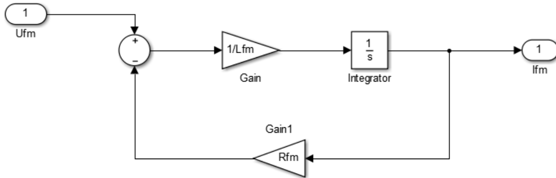
Slika 17. Model uzbudnog kruga motora izvedena u Simulinku
