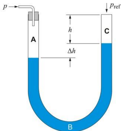
Slika 20. U-cijev [3]
