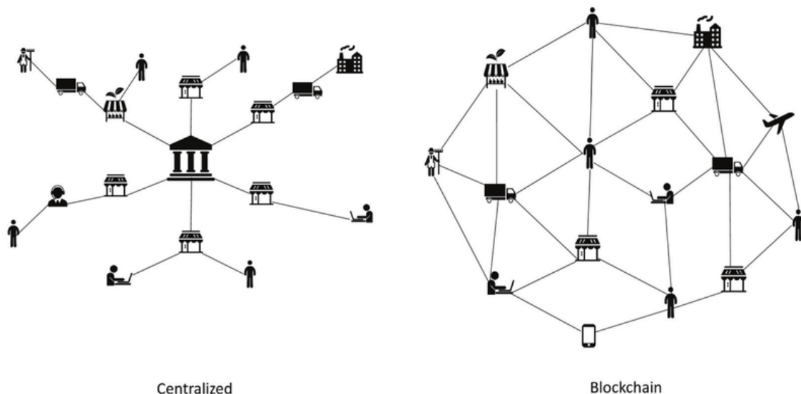
Slika 5. Decentralizacija blockchaine
