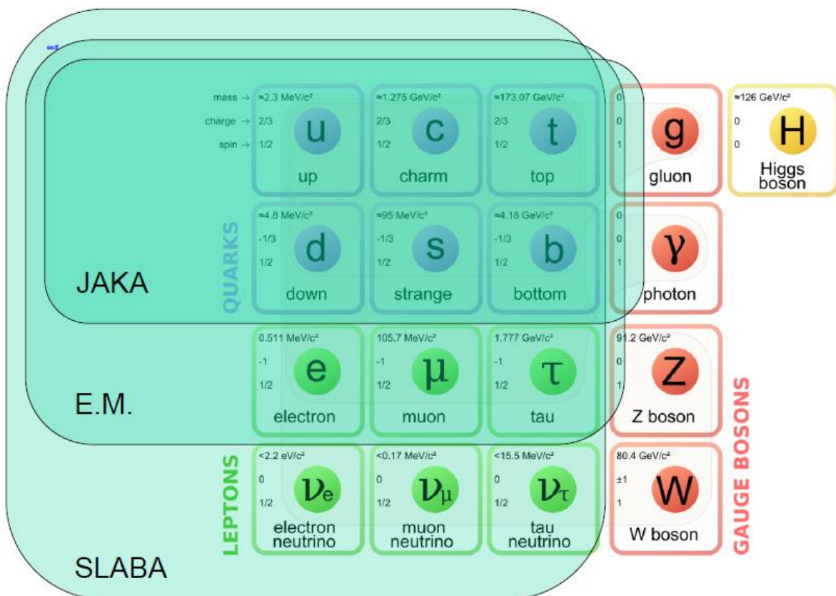
Slika 9: Čestice Standardnog modela i njihove interakcije [2]
