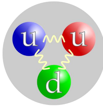
Slika 4: Struktura protona sastavljena od tri kvarka [16]
