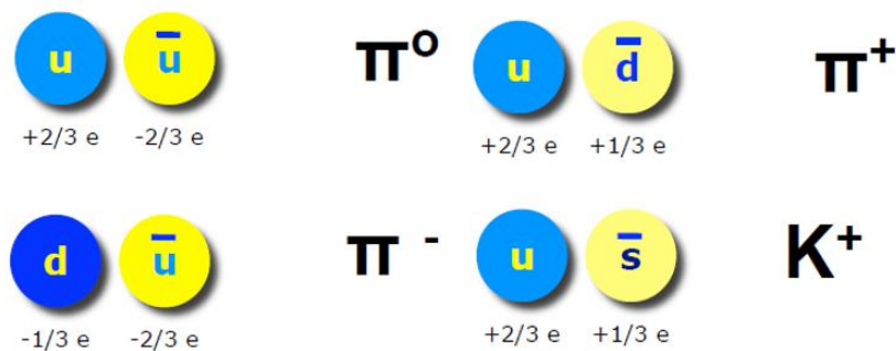
Slika 7: Par kvark-antikvark (pi-mezon i K mezon) [2]
