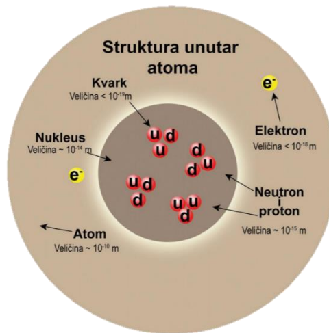
Slika 5: Struktura atoma [18]
