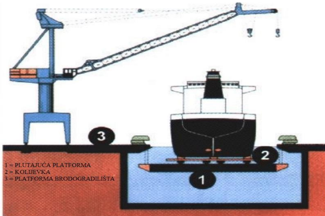
Slika 1. Oprema syncro-lifta [6]
