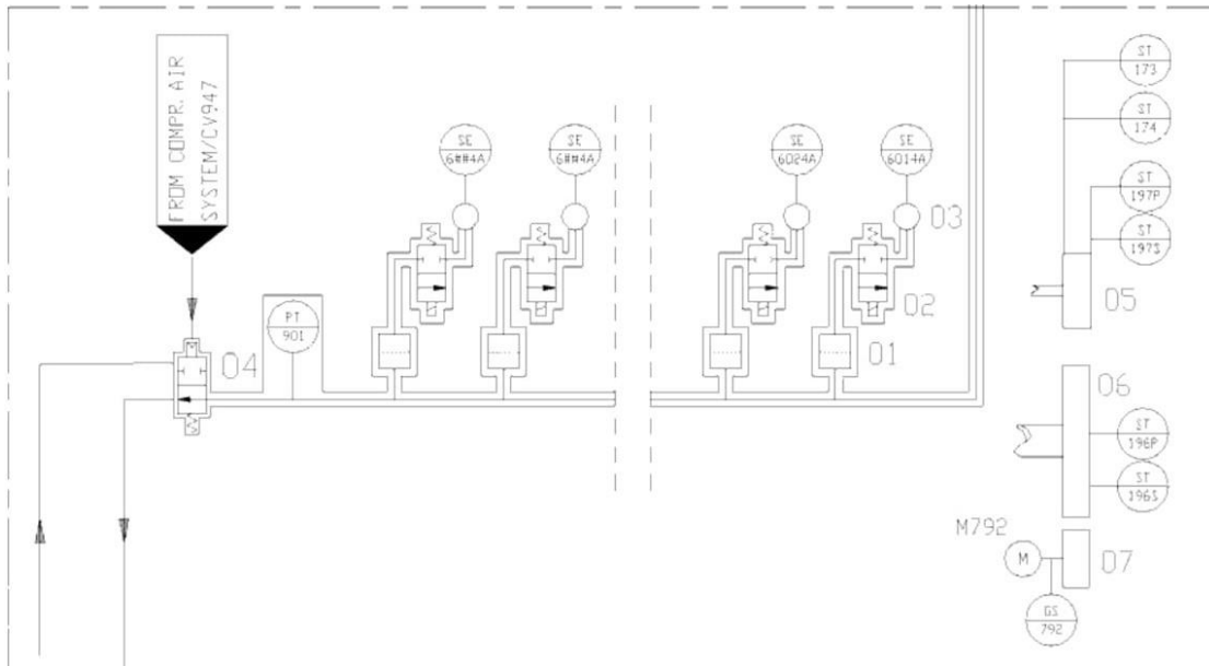
slika 8. Sustav plina [2]
