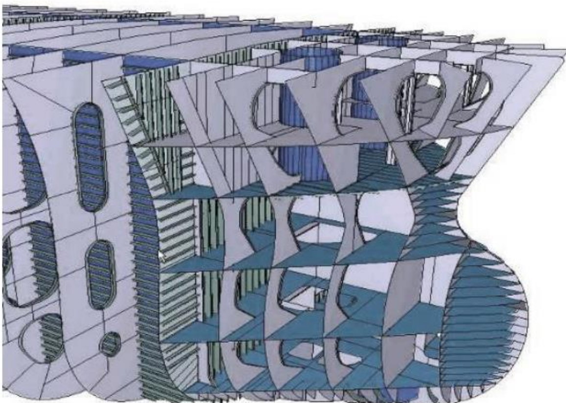
Slika 18. Kolizijske pregrade [13]
