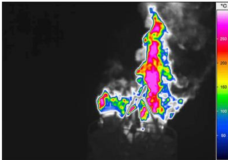
Slika 9. Termografski snimak plinske baklje [6]
