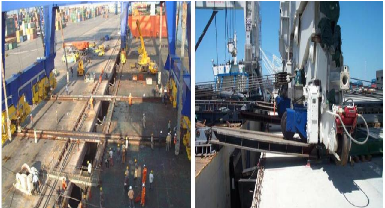
Slika 20. Razni oblici čeličnih greda za ukrcaj [4]
