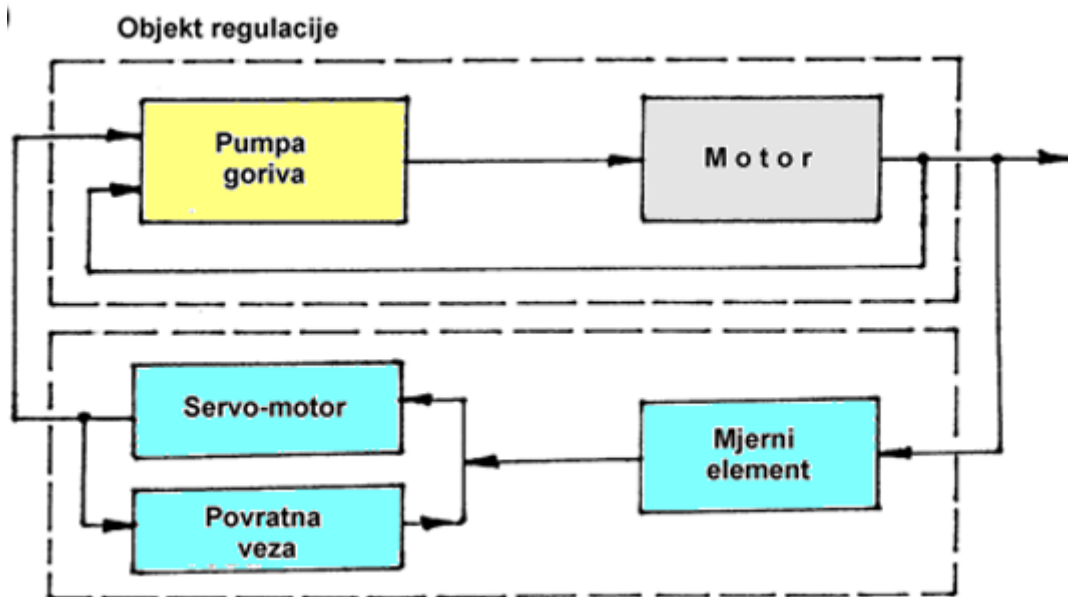
Slika 5. Strukturalna shema sustava automatske regulacije neizravnog djelovanja [6]
