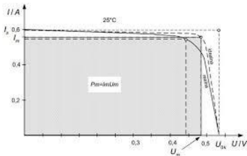
Slika 16. Maksimalna snaga sunčane ćelije [8]
