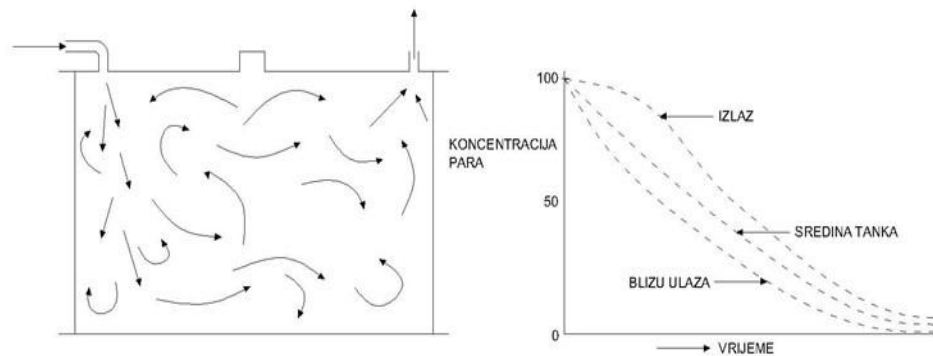
Slika 11. Inertiranje miješanjem [7]
