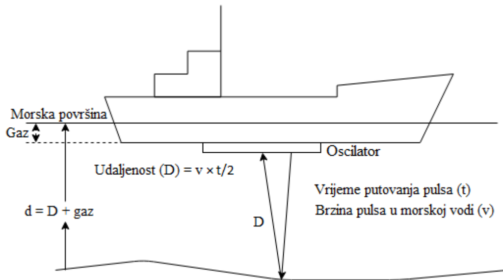
Slika 8. Princip rada ultrazvučnog dubinomjera [59]
