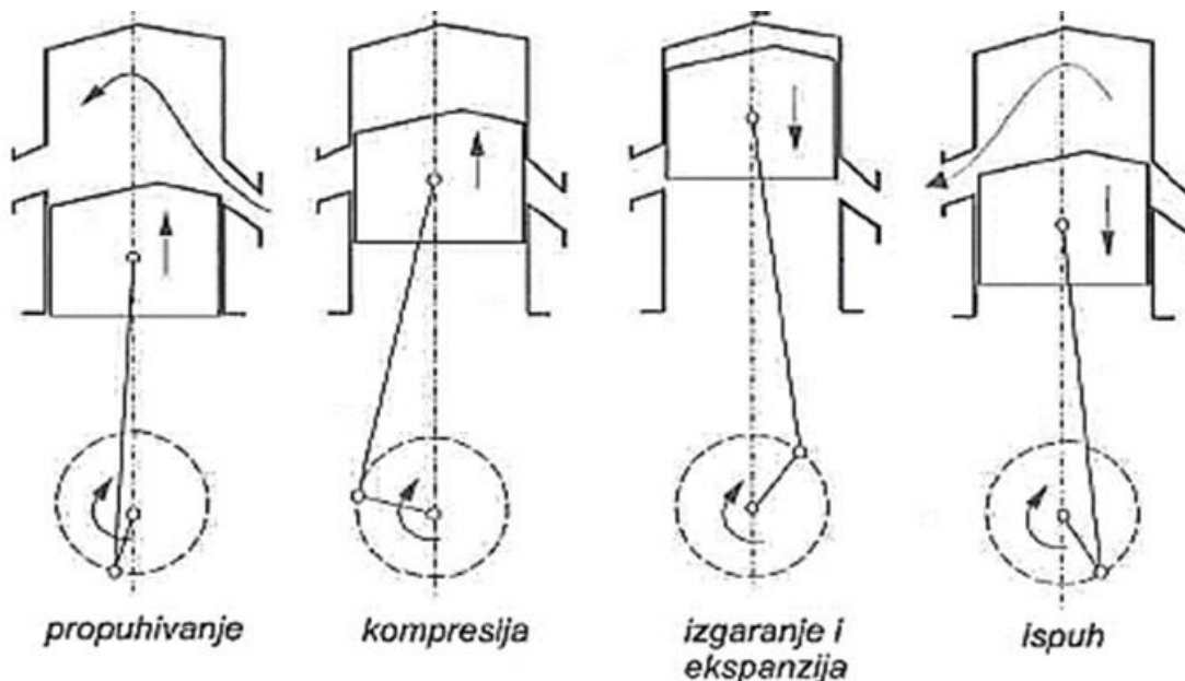
Slika 6.Taktovi 2T motora [7]
