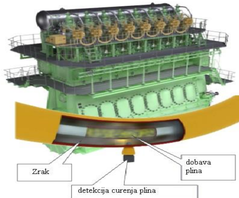
Slika 25. Sistem s dvostrukom stijenkom [17]
