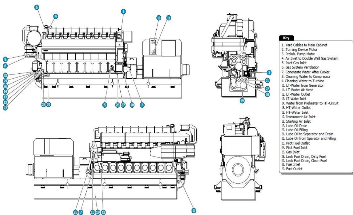
Slika 11. Wartsila 9L34DF [19]
