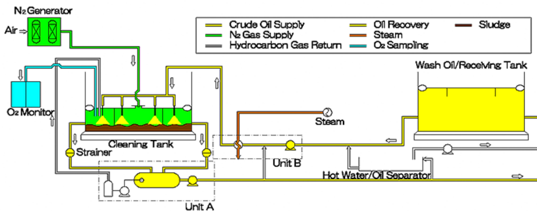
Slika 5. Sustav za pranje sirovom naftom [14]
