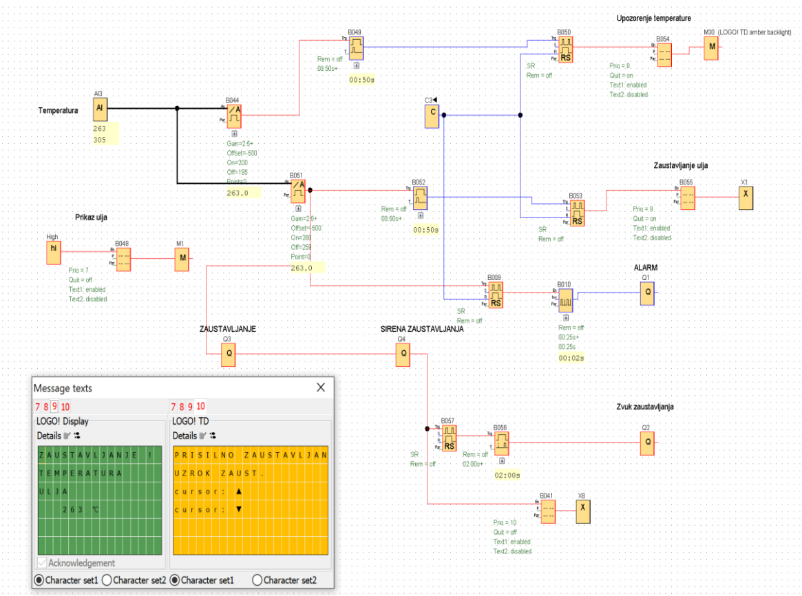
Slika 25 Shema automatiziranog sustava za nadzor temperature s interaktivnim ekranom, zaustavljanjem u nuđi i zvučnim signalima
