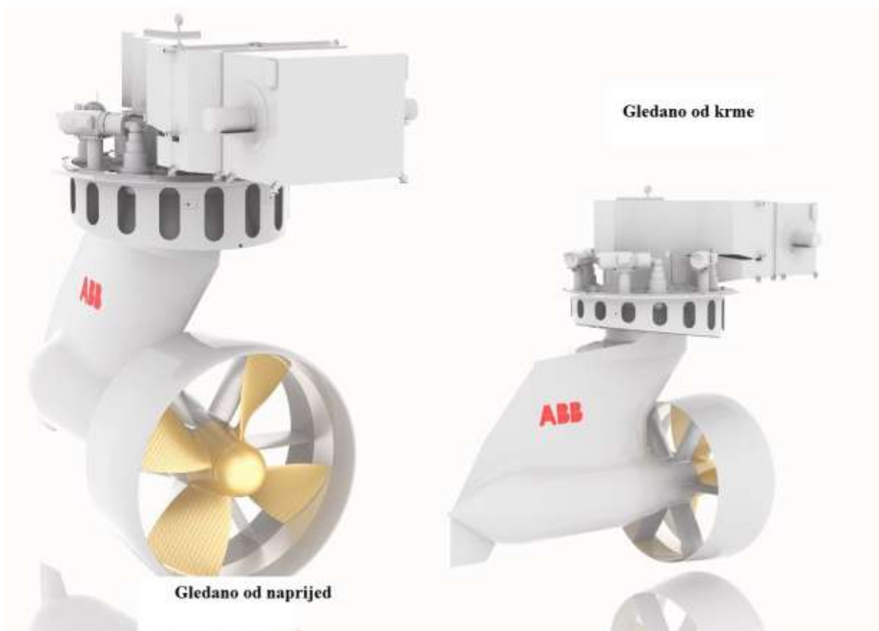
Slika 5. Pod-propulzor u sapnici [6]
