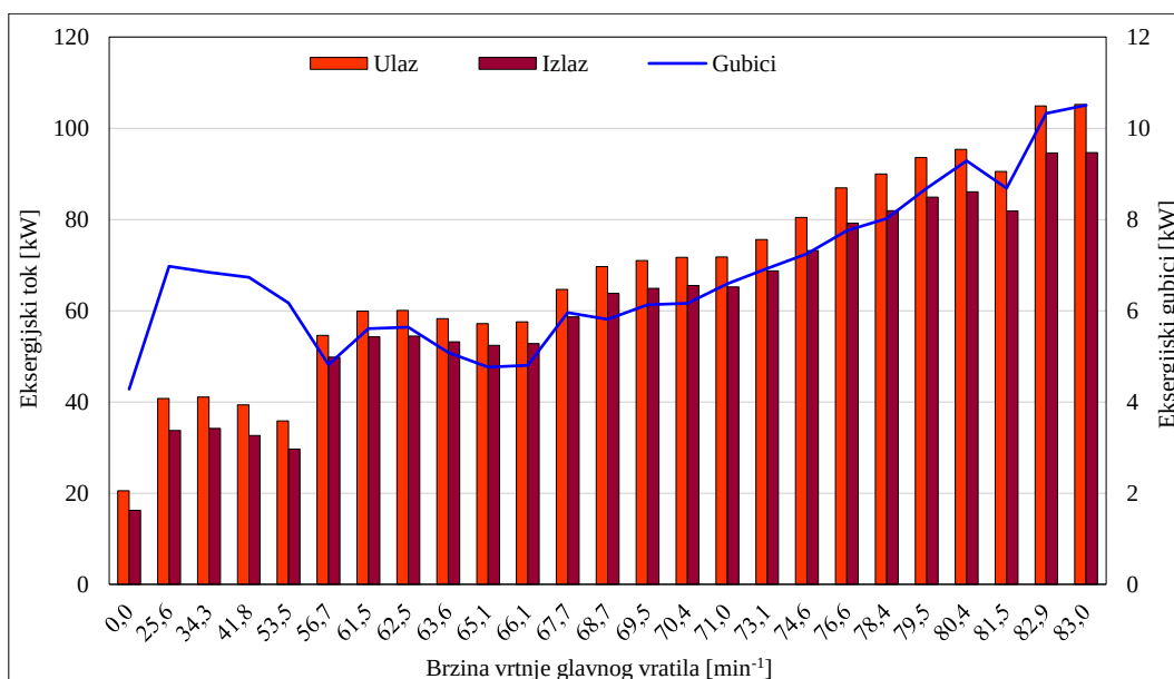
Slika 44. Kretanje eksergijskih tokova mlakog zdenaca pri promjeni opterećenja [37]
