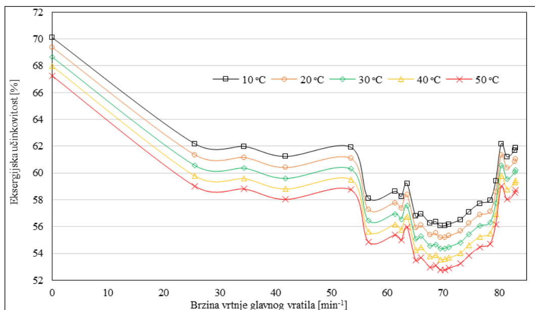
Slika 9. Kretanje eksergijske učinkovitosti turbogeneratora pri promjeni temperature okoline [37]
