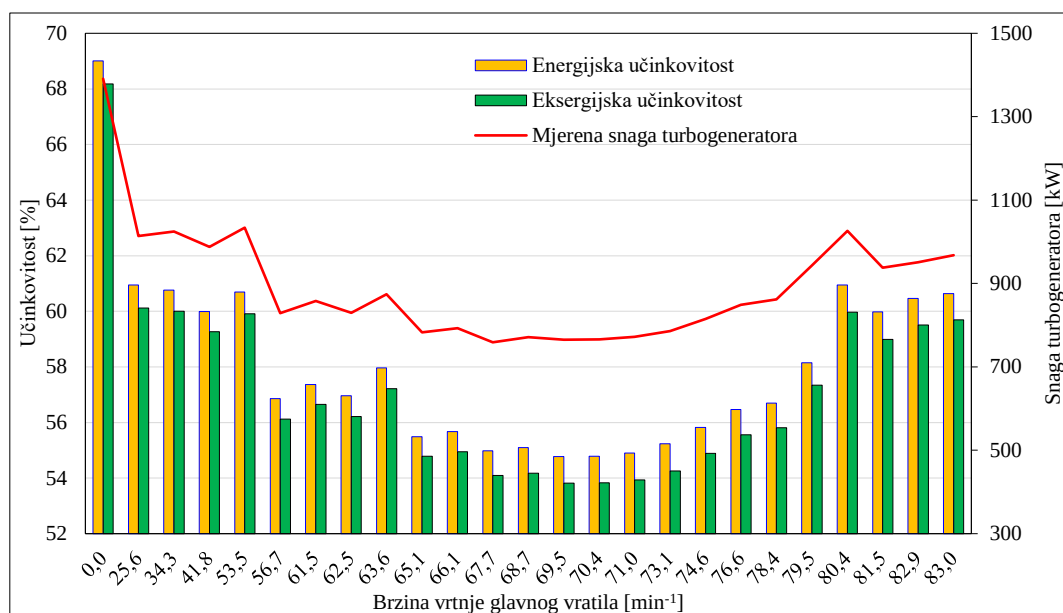
Slika 8. Energijska i eksergijska učinkovitost turbogeneratora u odnosu na mjerenu snagu pri promjeni opterećenja [37]
