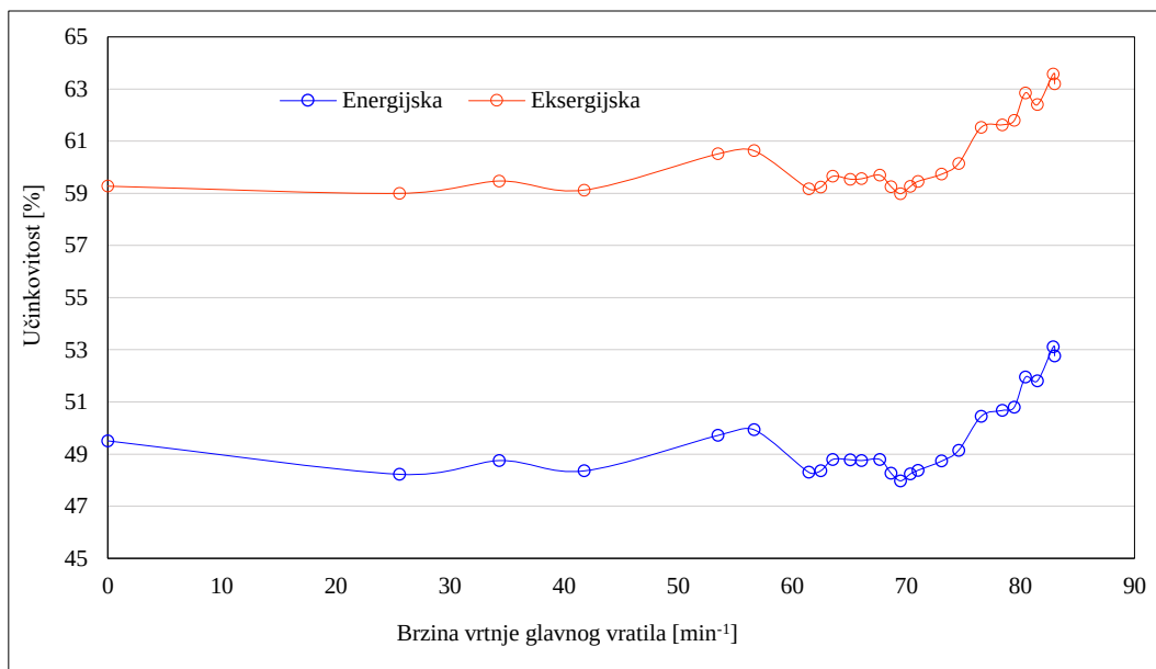
Slika 13. Energijaska i eksergijska učinkovitost turbine napojne pumpe pri promjeni opterećenja [37]
