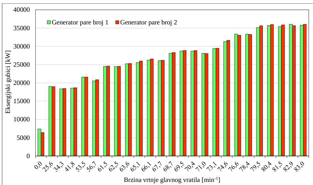
Slika 20. Eksergijski gubitci na generatorima pare pri promjeni opterećenja [37]
