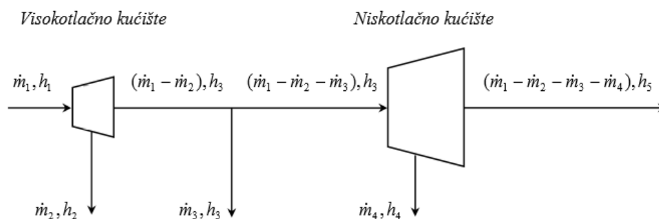
Slika 4. Termodinamički model brodske parne turbine [37]
