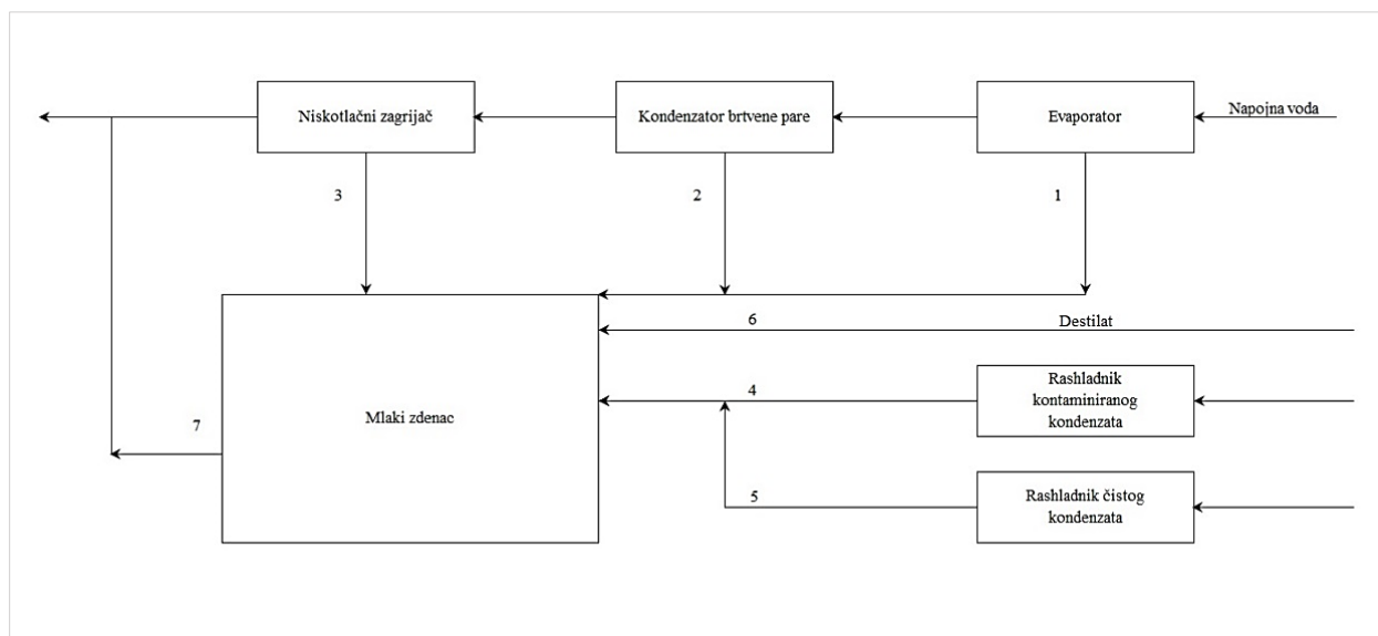
Slika 41. Sustav napojne vode i mlaki zdenac [37]
