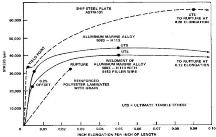
Slika 24. Krivulja naprezanja – deformacije za Aluminijску slitinu 5083 [37]
