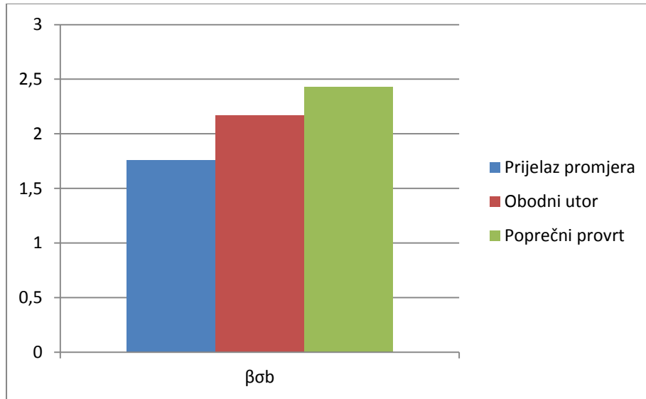
Slika 15: Usporedba efektnog koeficijenta koncentracije naprežanja na savijanje za karakteristične presjeke
