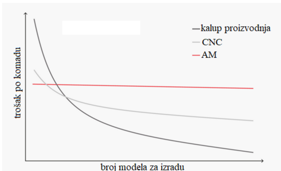
Slika 11. Dijagram ekonomije tehnologije izrade modela[1]
