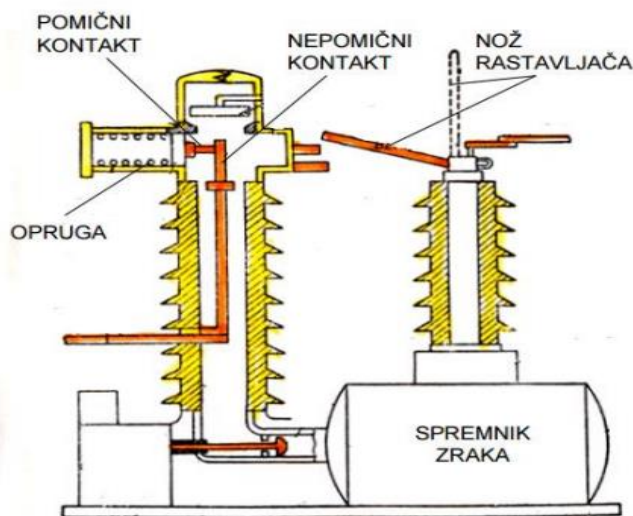
Slika 21. Zračni prekidač [14]
