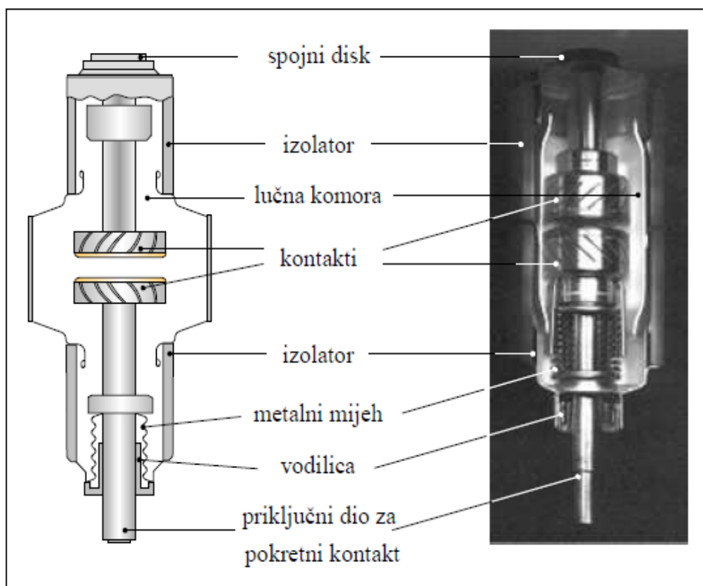
Slika 22. Vakuumski prekidač [14]
