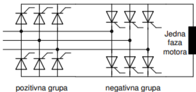
Slika 26. Ciklokonverter [16]
