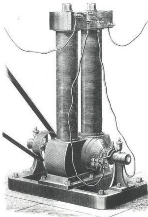
Slika 4. Edisonov dinamo [1]
