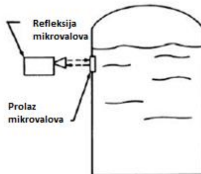
Slika 23. Radarski senzor razine [2]
