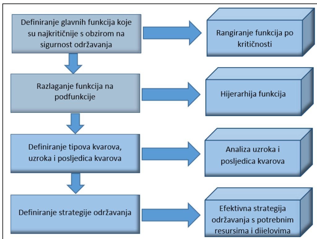
Slika 7. RCM metodologija
