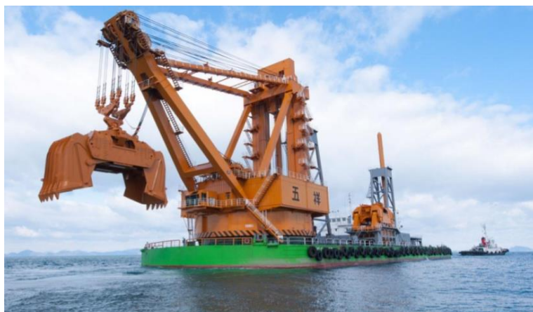
Slika 36. GOSHO, jaružalo s najvećom grabilicom od 200 m 3 [34]
