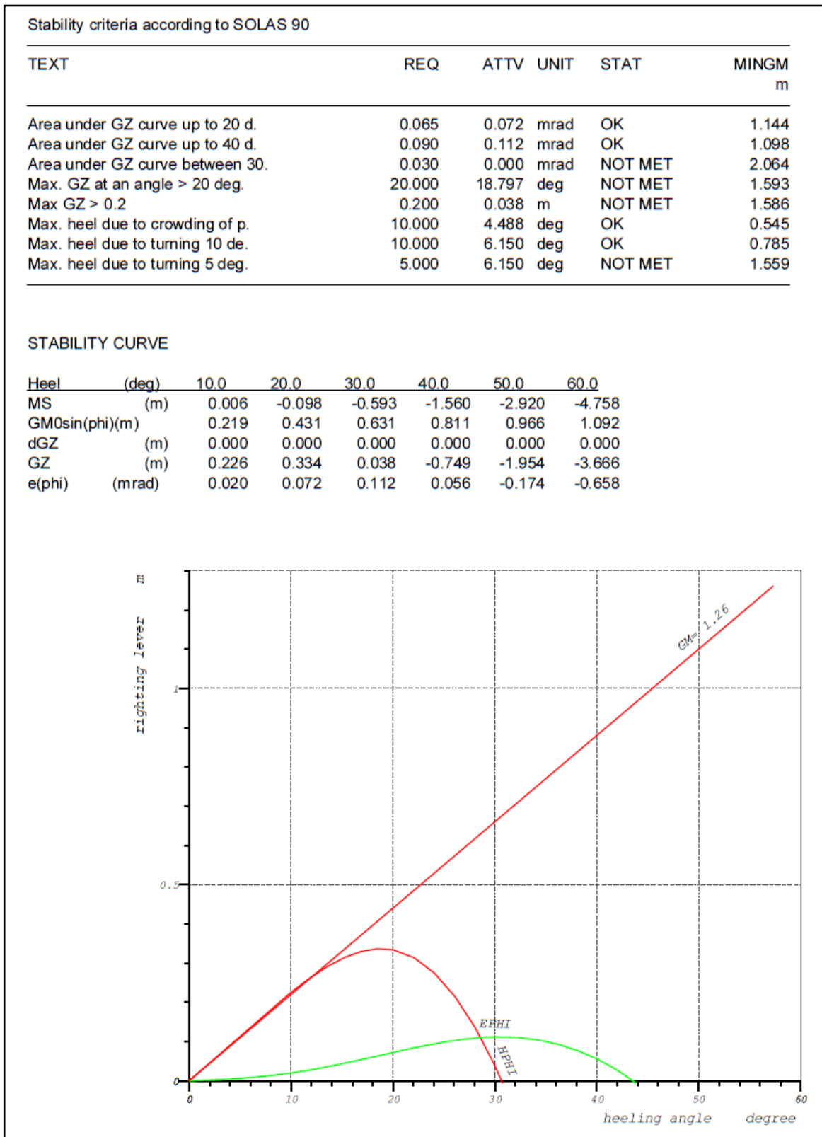
Slika 11: Isječak iz HT-a, kriteriji stabiliteta u neoštećenom stanju
