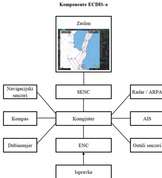
Slika 4. Komponente ECDIS-a [9]
