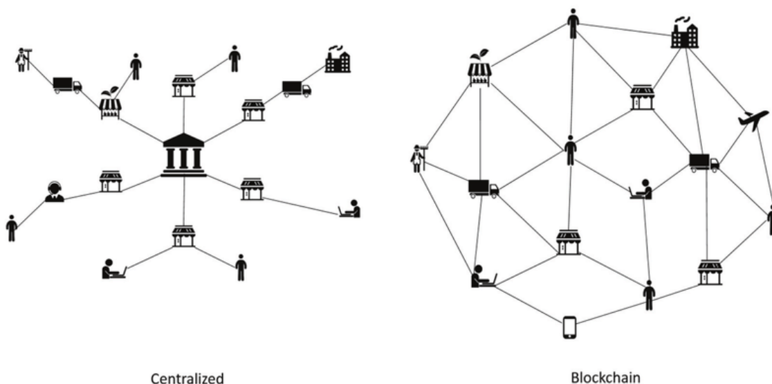
Slika 5. Decentralizacija blockchaine
