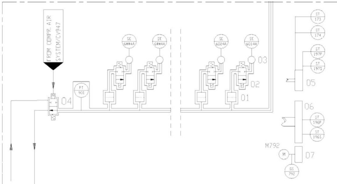
slika 8. Sustav plina [2]
