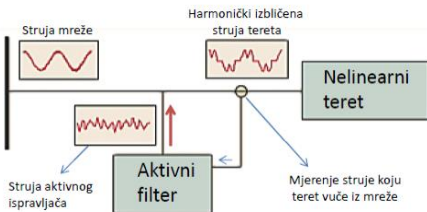
Slika 18. Princip rada aktivnog filtera [5]
