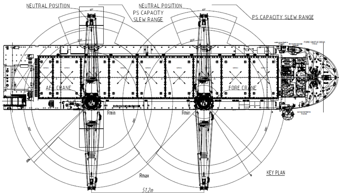
Slika 62. Sustav grotlenih poklopaca međupalube [2]
