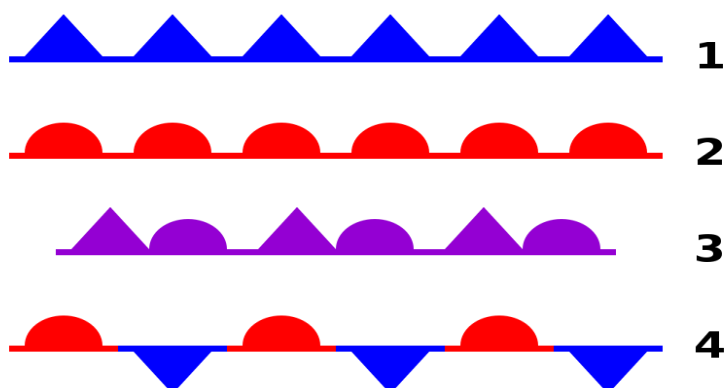
Slika 1. Simboli za atmosferske fronte: 1 hladna fronta; 2 topla fronta; 3 okludirana fronta; 4 stacionarna fronta [2].
